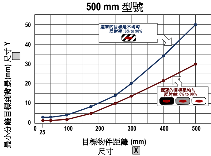
圖 12 最小物件間隔距離 (90% to 6% 反射)
